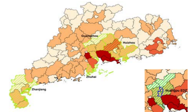
广东省各行政区域的光伏发电技术潜力（颜色越深，潜力越大）
