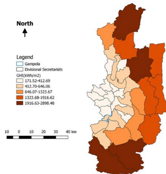
斯里兰卡中部省太阳能地图 (GHI为地面接受的太阳能辐射量)
